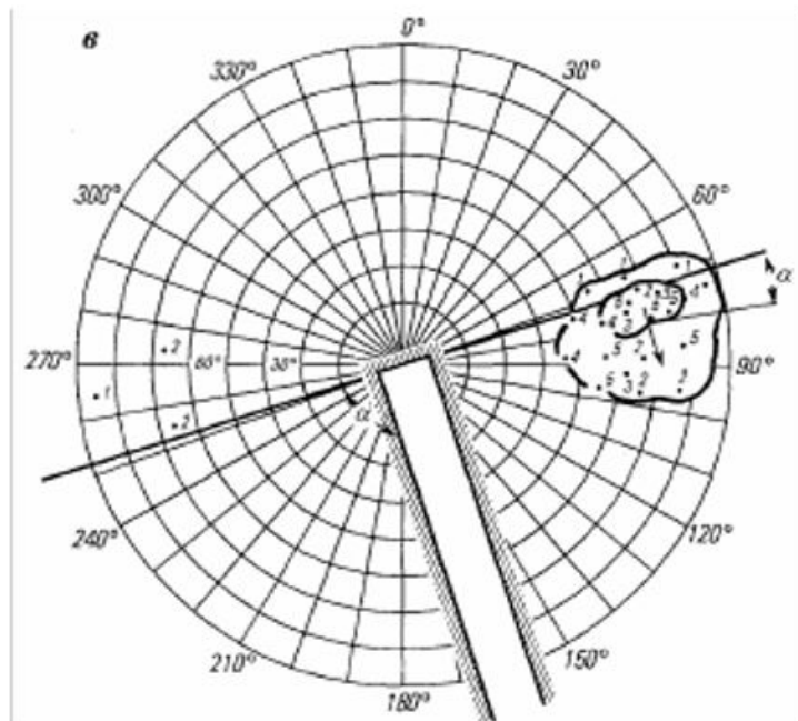
Рисунок 6. Ориентировка трещин относительно обнажения выработки: а - разрез, б - план, в - круговая диаграмма, \alpha - угол встречи трещины с обнажением
