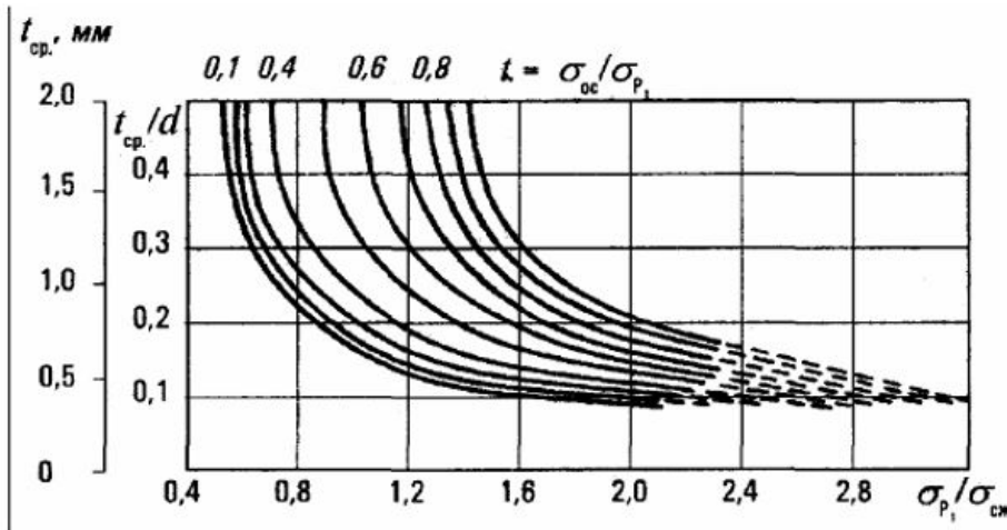
Рисунок 1. Зависимости параметров дискования керна t_{ср}/d_{диск} от уровня напряженности массива \sigma_{p1} / \sigma_{сж} при различных соотношениях между осевыми и радиальными напряжениями \sigma_{ос} / \sigma_{p1} : d_{диск} – диаметр дисков, t_{ср} – средняя толщина дисков
