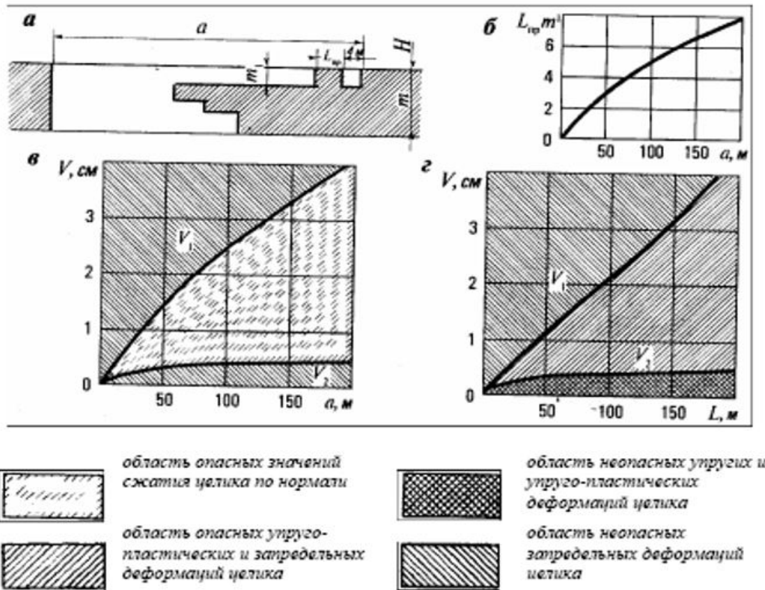
Рисунок 2. Оценка состояния податливых целиков: а - расчетная схема, б - зависимость предельного размера целика от ширины выработанного пространства, в - зависимость величины сжатия целика по нормали от ширины выработанного пространства, г - номограмма для оценки состояния целика по величине сжатия по нормали, m^1 – вынимаемая мощность слоя, Н – глубина разработки
