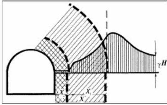
Рисунок 3. Схема, иллюстрирующая положение зоны дискования X_1 , X – расстояние от обнажения до зоны максимума опорного давления; X_1 = X - X_2 ; \gamma – удельный вес породы, H – глубина разработки
