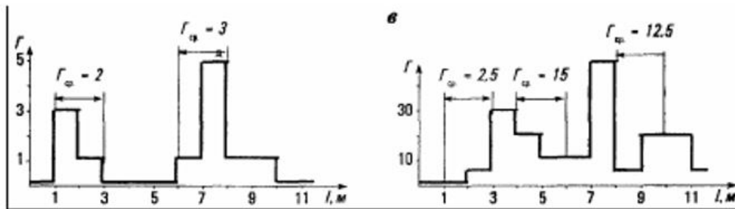
Рисунок 5. Определение интенсивности трещин: а - определение густоты (числа) трещин; б, в - примеры оценки средней густоты (числа). \Gamma_{ср} трещин поперечной направленности по длине участка выработки 1
